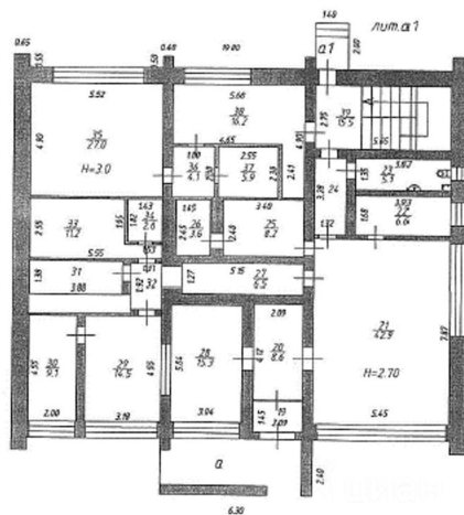
Позтажный план (1 этаж)
