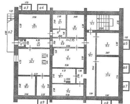
Позтажный план (подвал)
